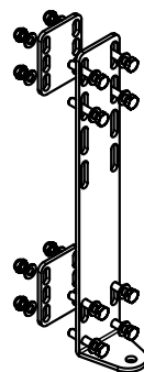
Pletina de fijación inferior. Eje entre los escalones 250\text{mm} < e < 400\text{mm}
