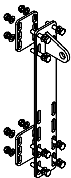
Pletina de fijación superior. Eje entre los escalones 250\text{mm} < e < 400\text{mm}
