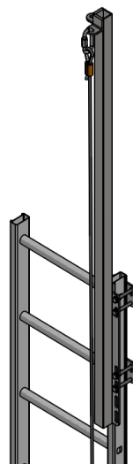
Prolunga con fissaggio su corrimano laterale Altezza 1500mm
