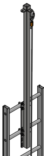
Prolunga con fissaggio su piolo Altezza 1500 mm
