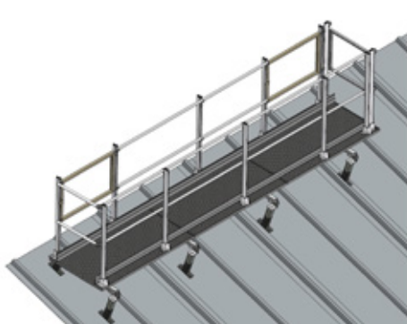
Pasarela sobre cubierta Zinc chilla
