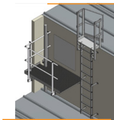
Pasarela sobre paramento vertical
