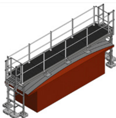
Pasarela sobre chapa perfilada
